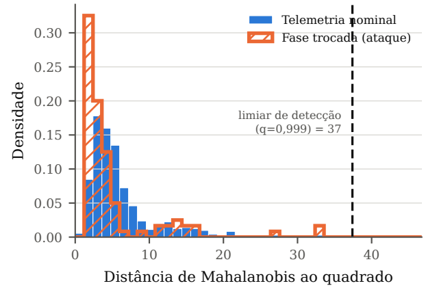
Figura 5. Distribuições de escore sob a sonda de troca de fase. Quadros de bordo reproduzidos de meia órbita antes situam-se dentro, e de fato abaixo, da distribuição nominal, porque a fase orbital é marginalizada por uma linha de base ajustada sobre uma órbita inteira. A textura é redundante com a cor, para impressão em tons de cinza.
