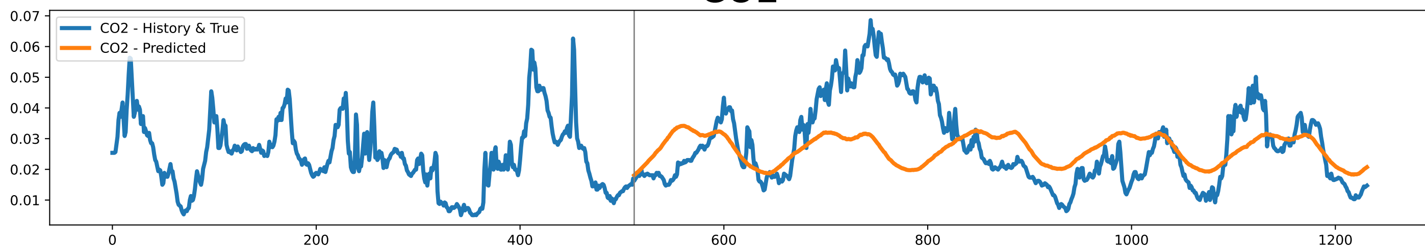
CO2
