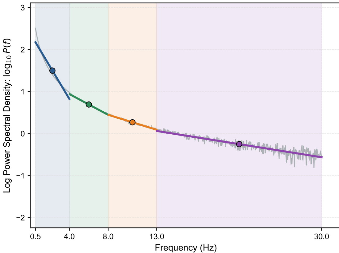
Non-Seizure EEG
