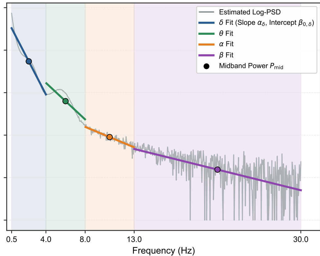
Seizure EEG
