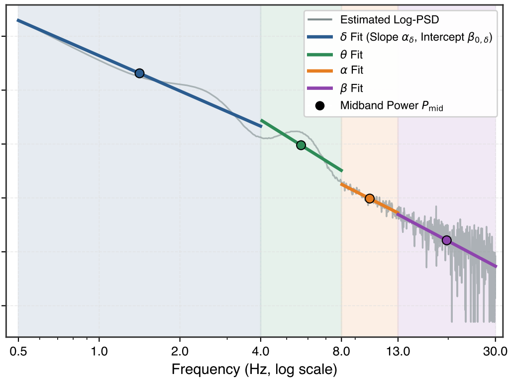
Ictal Neonatal Seizure EEG
