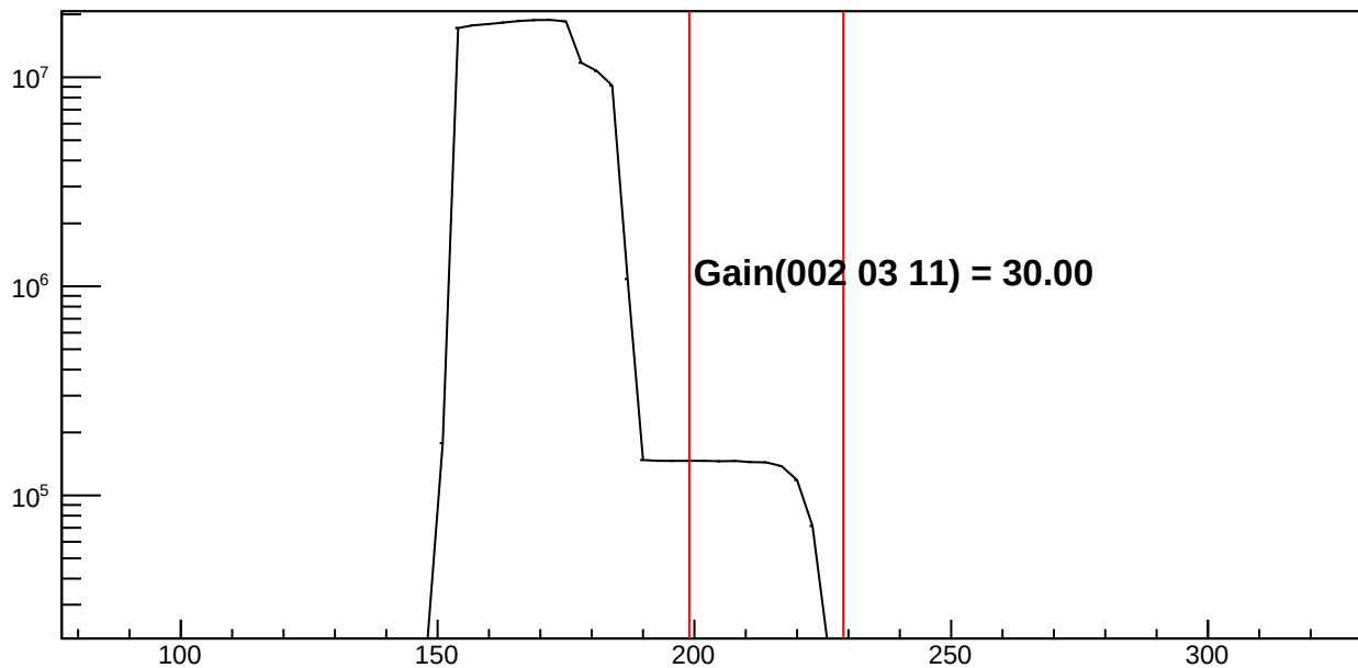
Log Transformed Y Values Histogram
