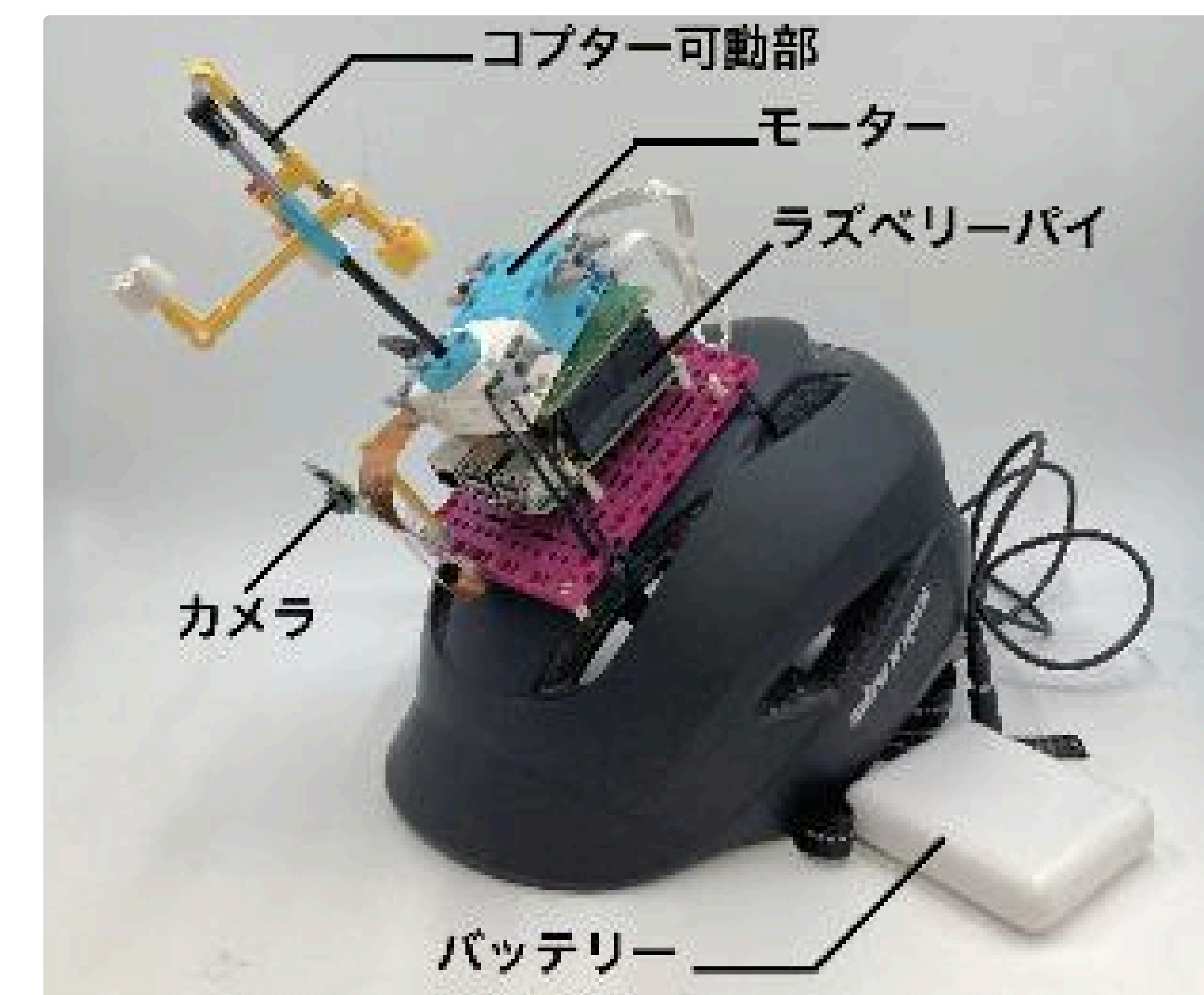
コプター構成図
