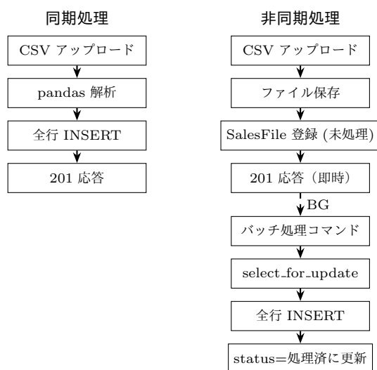
図 3 同期・非同期 CSV 処理フロー比較
