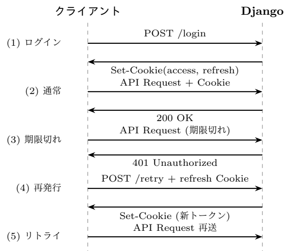
図 2 JWT 認証フロー
