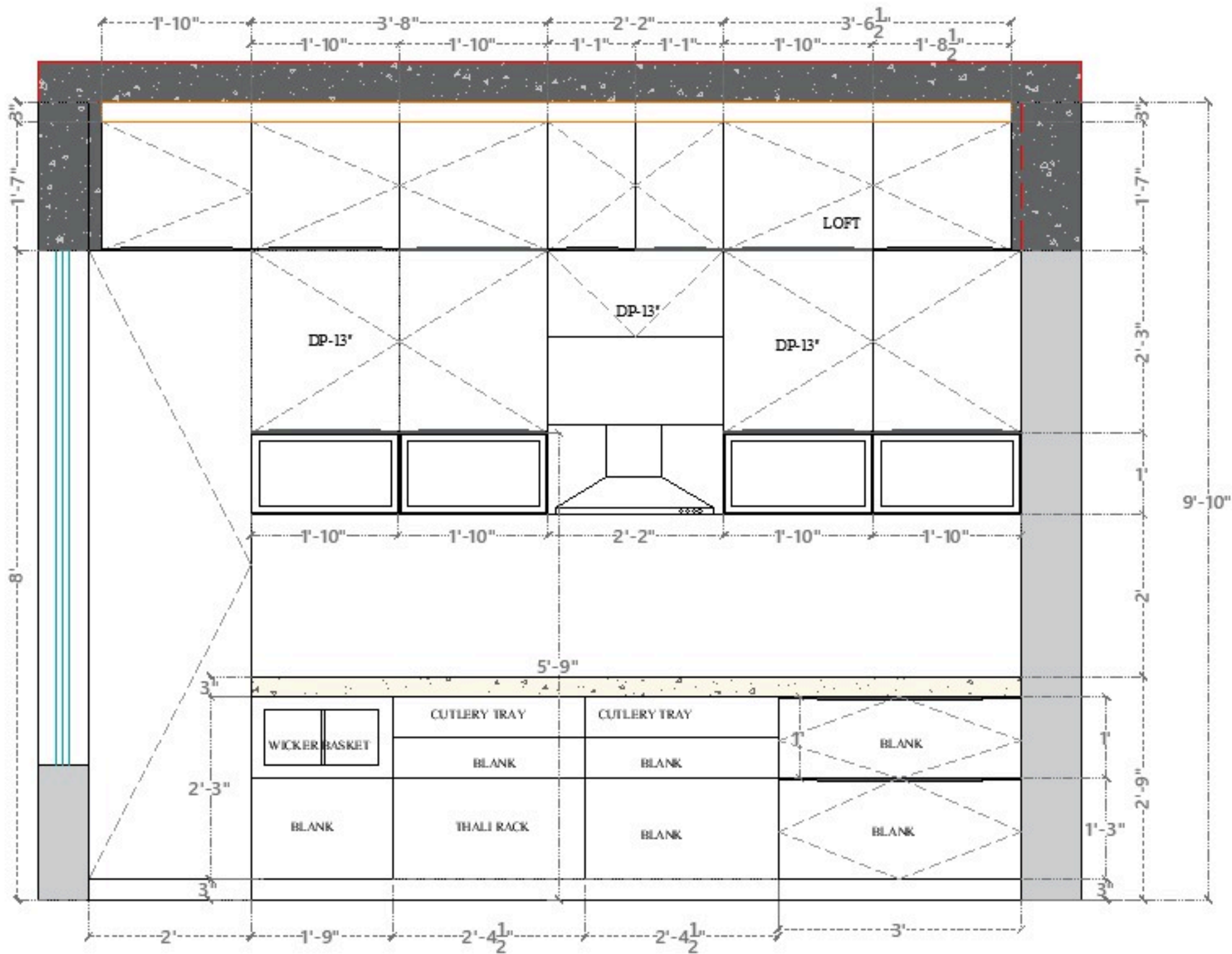
ELEVATION -A
