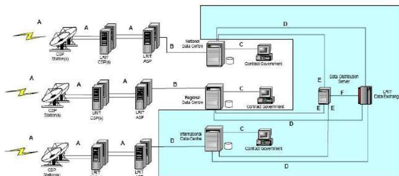
FIGURA 3 - COMPONENTES DO SISTEMA DE COMUNICAÇÃO LRIT
