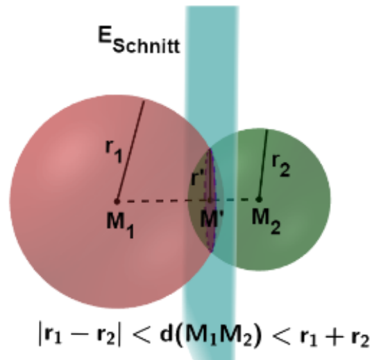
Abbildung 2: Kollision der zwei Kugeln [2]
