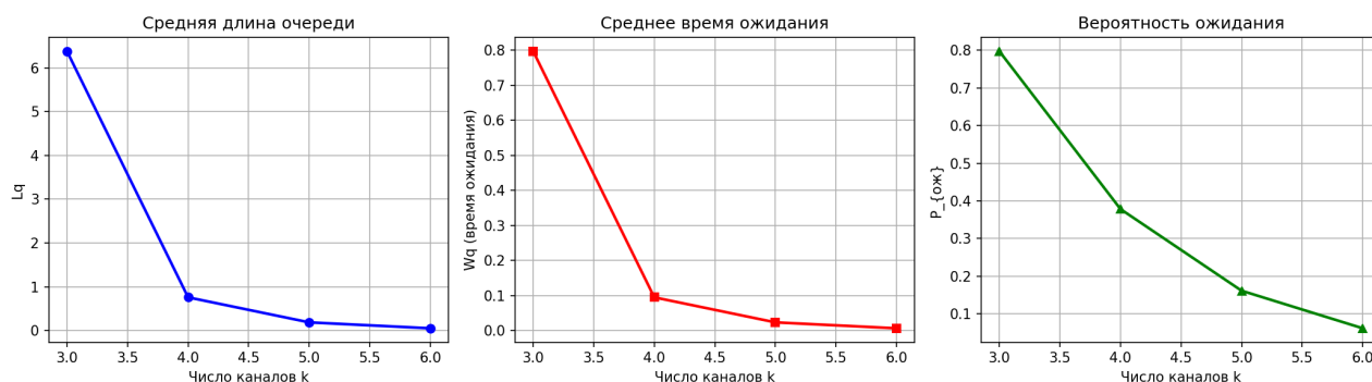
Рисунок 3.1 – Зависимость L_q , W_q и P_{\text{ож}} от числа каналов k при \lambda = 8 , \mu = 3
