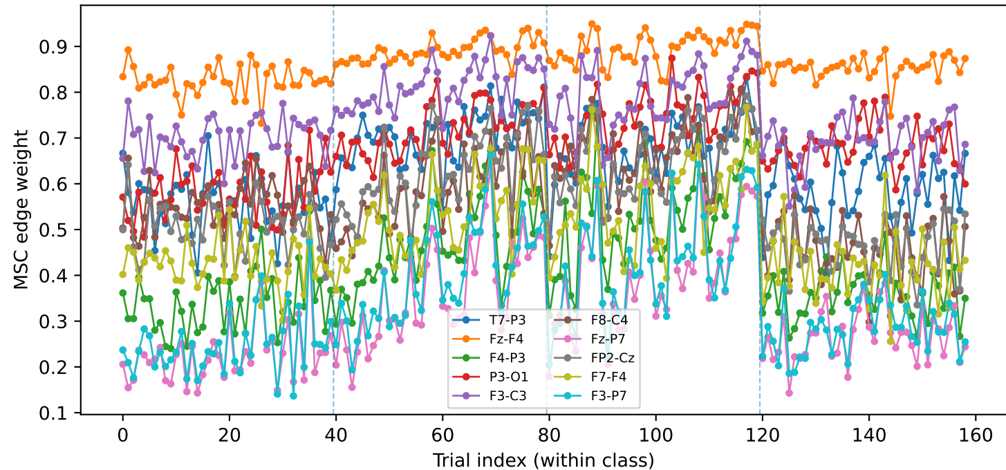
S31 MSC - Top-KL edge trajectories (L)
