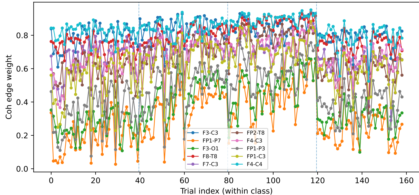
S31 Coh - Top-KL edge trajectories (R)
