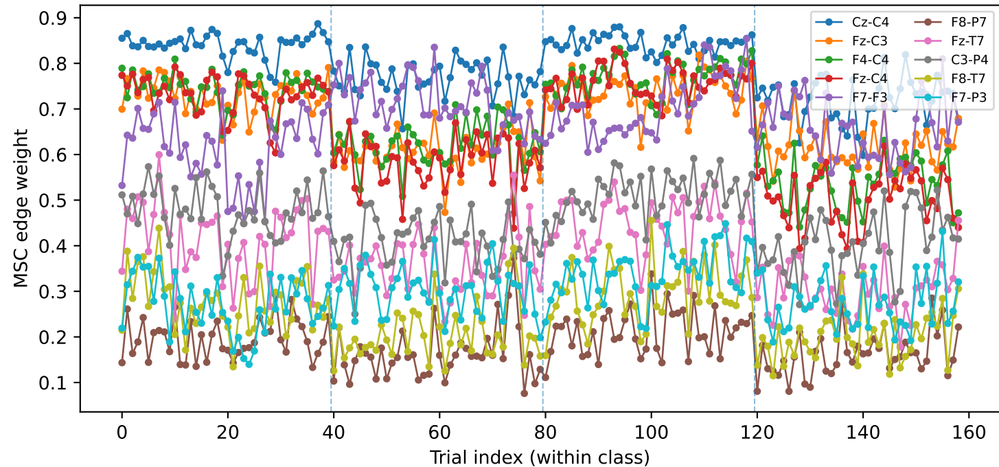
S21 MSC - Top-KL edge trajectories (L)
