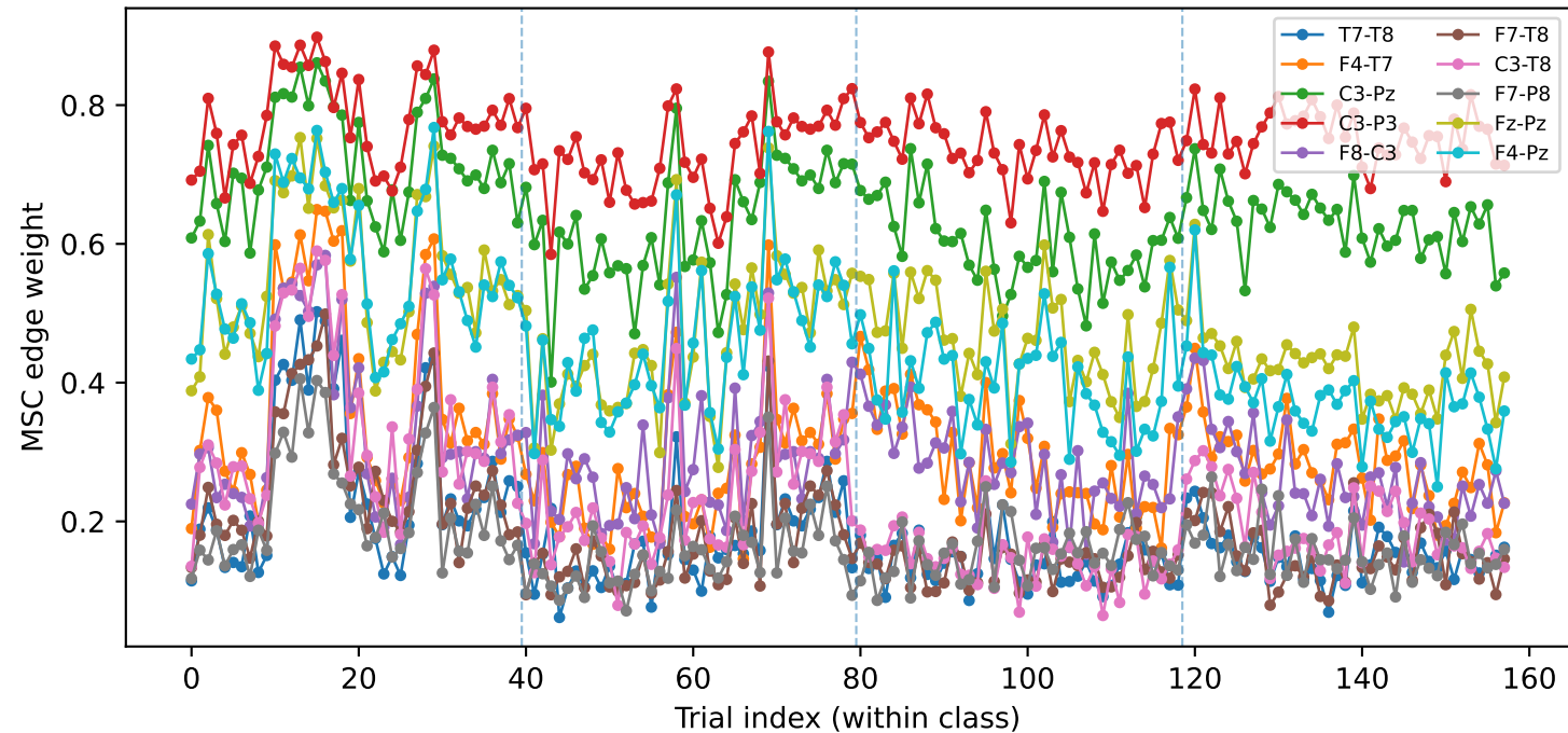
S09 MSC - Top-KL edge trajectories (R)
