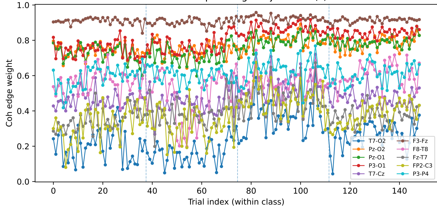
S34 Coh - Top-KL edge trajectories (L)
