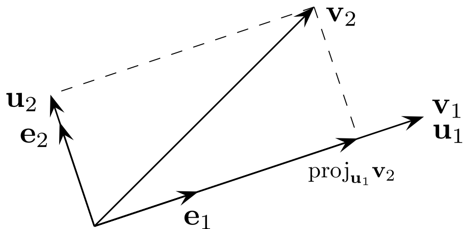
Schema del processo di Gram-Schmidt
