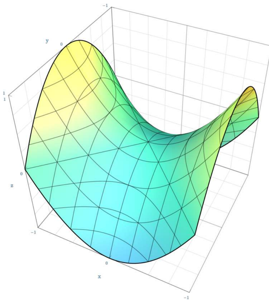
Paraboloide iperbolico
