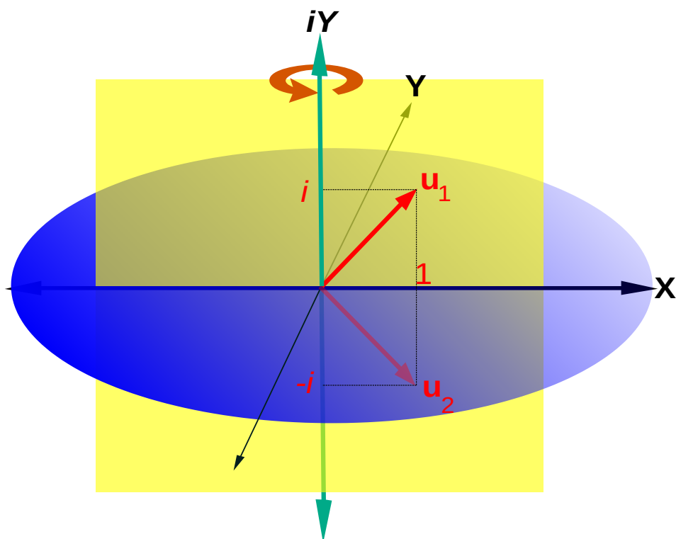
Autovettori in una rotazione
