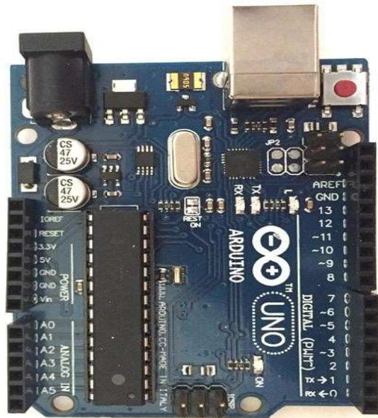
Fig3.2 ARDUINO UNO
