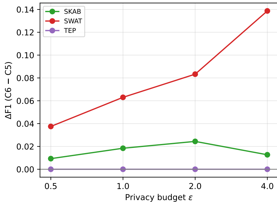
\Delta F1 vs \epsilon by dataset
