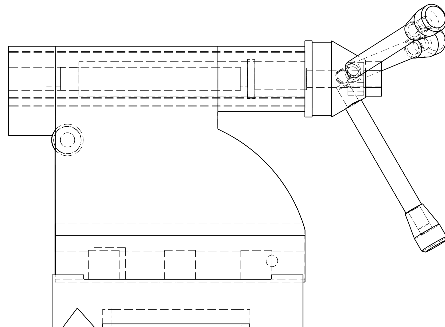
Left view Scale: 2:3
