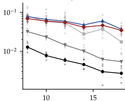
Erdős-Rényi G(N, 0.3)
