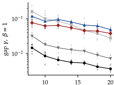
unit-disk
