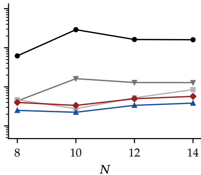
Erdős-Rényi G(N, 0.3)
