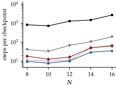
unit-disk
