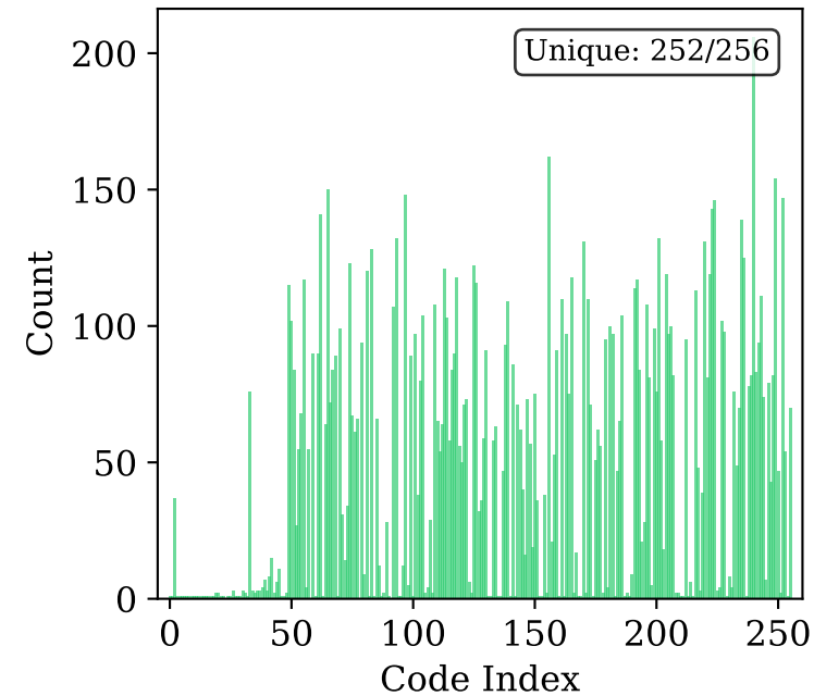
CSJ-ID Level 4
