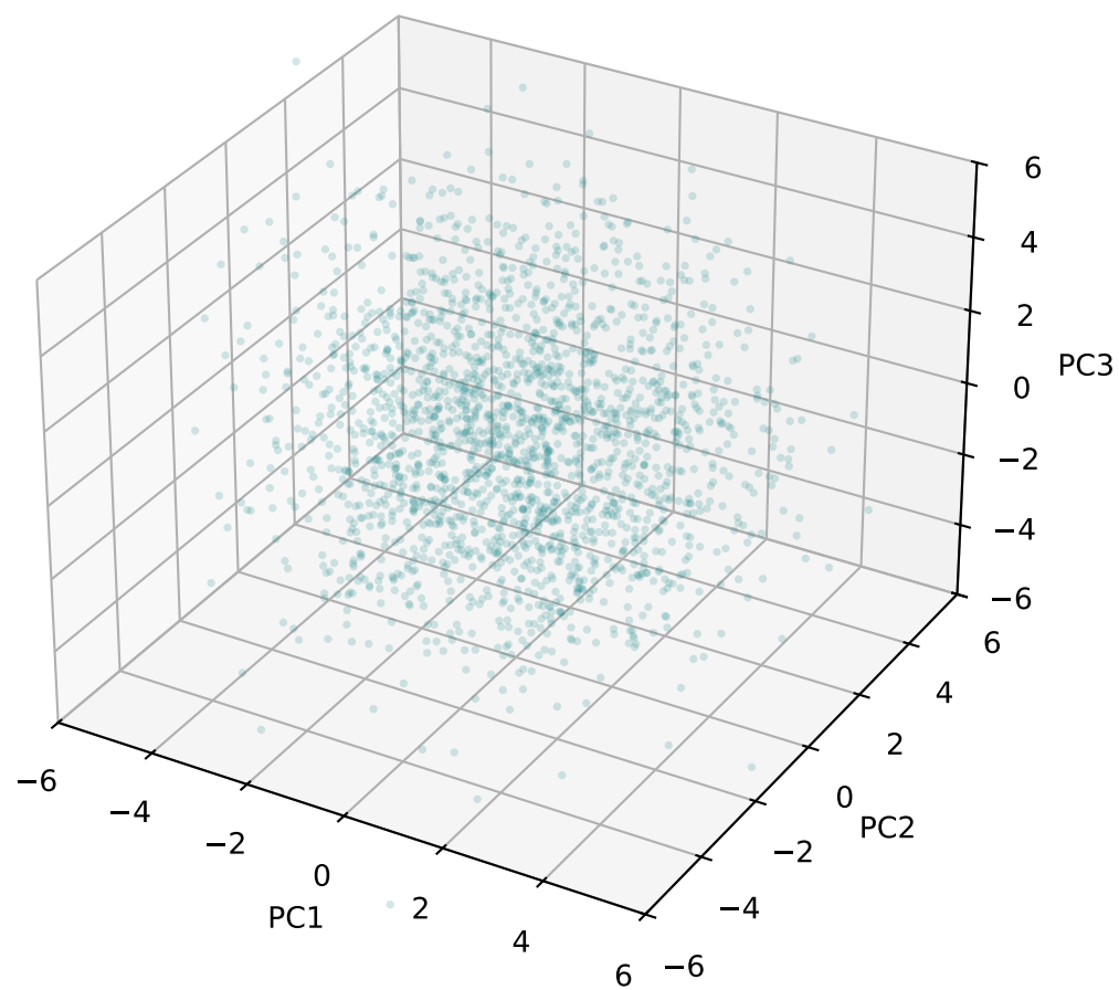
gauss \sigma=1
