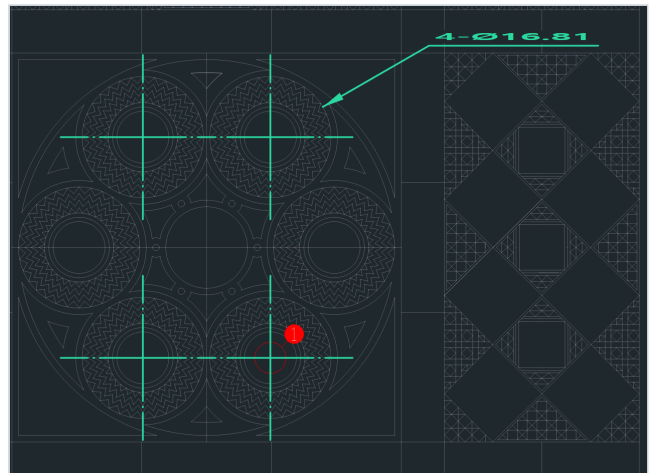
[그림 14-2] 수정 예시 표시 — 같은 지름 구멍 4개를 4-Ø16.81로 묶어 한 번만 기입하고 중심 마크 4개를 겹쳐 표시하였다.
