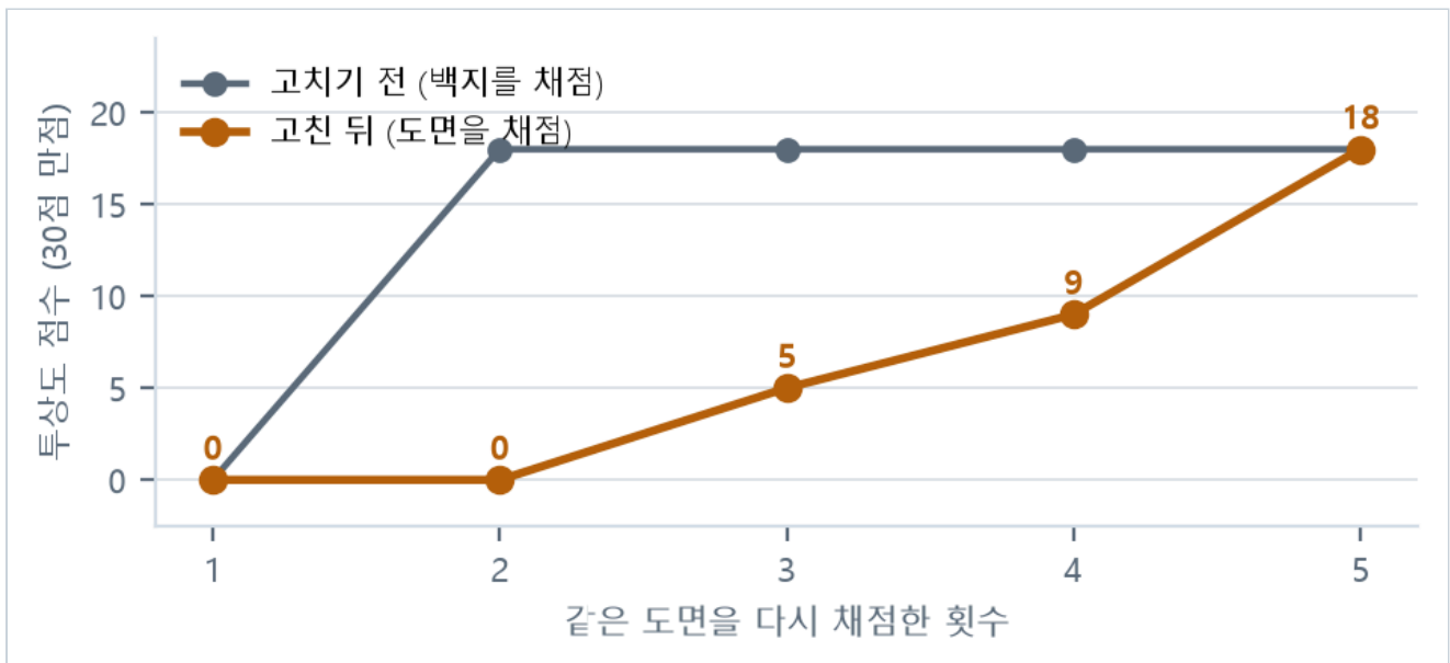
[그림 7] 백지 렌더링 조치 전후의 점수 분포 (sample_075em07z.dwg, 5회). 편차는 줄지 않았다. 오히려 점수 중앙값이 18점에서 5점으로 하락하였고, 지적 건수도 1건에서 1~3건으로 흔들리기 시작하였다.
