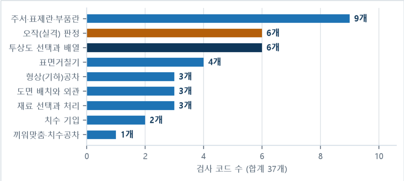
[그림 3] 검사 항목 37종의 분류별 개수. 주서·표제란·부품란이 9종으로 가장 많은데, 이는 확인 대상이 문자 기반이어서 규칙으로 판정 가능한 항목이 많기 때문이다. 반대로 투상도 6종 중 1종( AI_PROJECTION )은 규칙으로 판정할 수 없어 AI에 위임한다.
