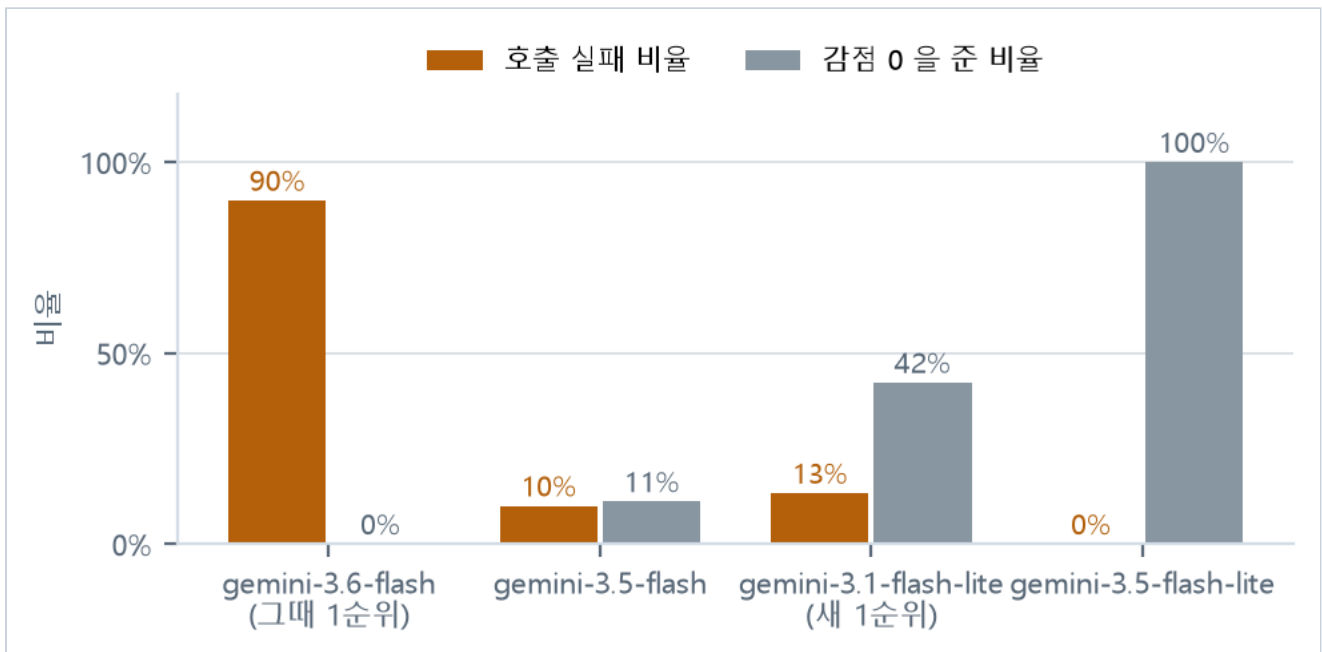
[그림 4] 채점 모델별 호출 실패 비율과 "감점 0"을 부여한 비율. 속도만으로 선정하지 않았다. 가장 빠른 gemini-3.5-flash-lite 는 20회 전부 감점 0을 부여하여 무엇을 입력하든 만점을 주는 상태였으므로 채택하지 않았다.
