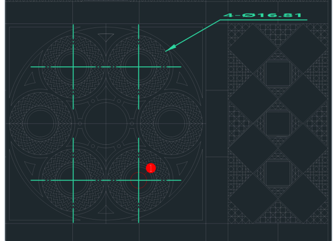
그림 9. 수정 예시 를 컨 화면. 같은 지름 구멍 4개를 4-Ø16.81 로 묶어 한 번만 적고, 중심 마크 4개를 초록색으로 얹었다. 실제 서비스 출력을 그대로 캡처한 것이다.
