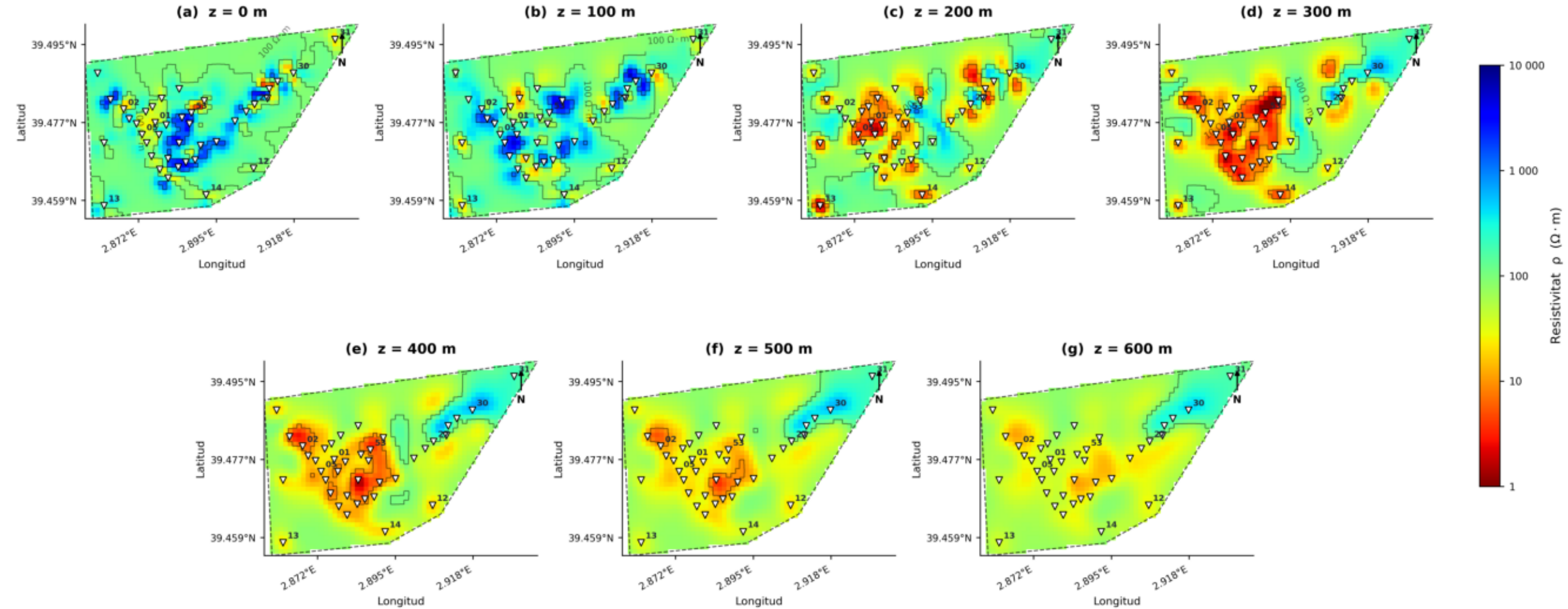
Model de resistivitat magnetotel·lúrica 3-D de la zona de Lluçmajor (Mallorca) — talls horitzontals de profunditat
