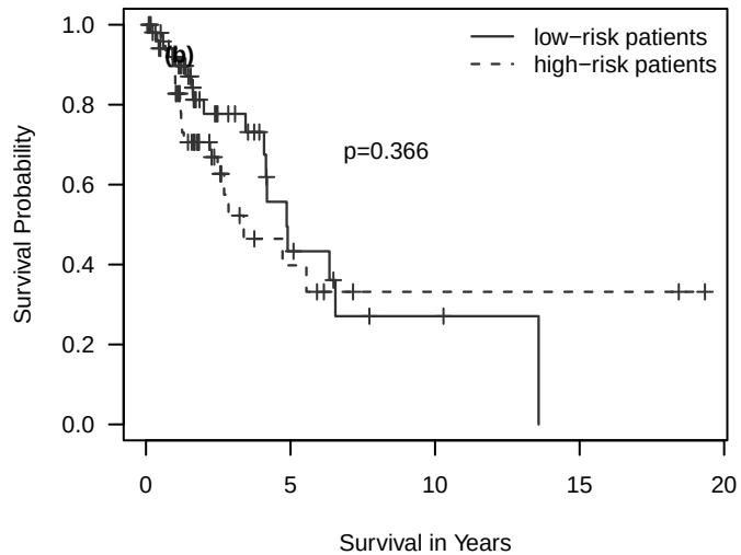
ContiCox
