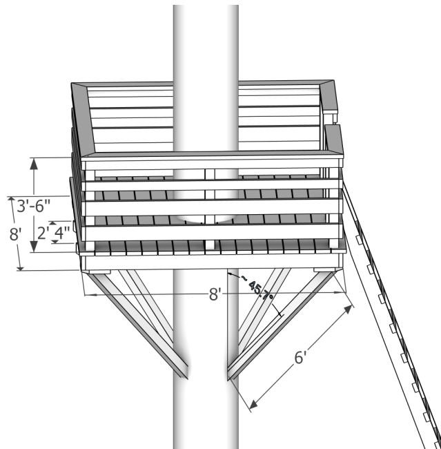
Fig. 3 - Dimensions
