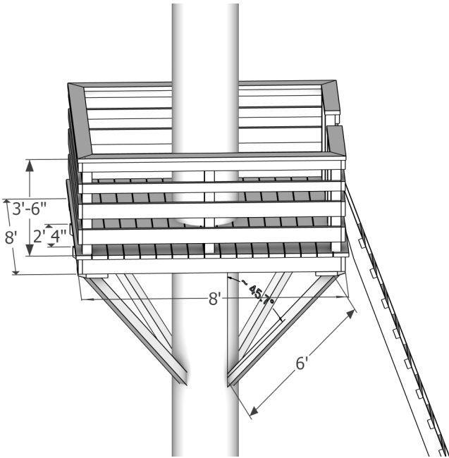
Fig. 2.2 - Dimensions
