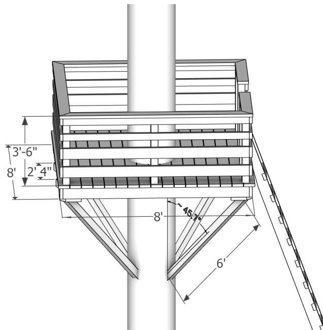
Fig. 3 - Dimensions
