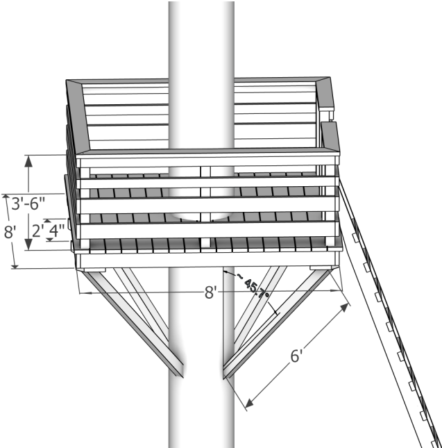
Fig. 3 - Dimensions
