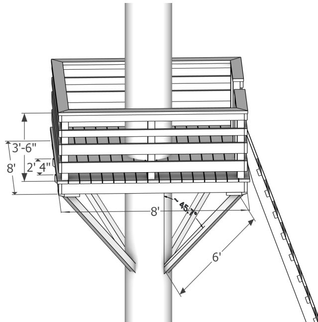
Fig. 3 - Dimensions
