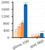
Faiss
