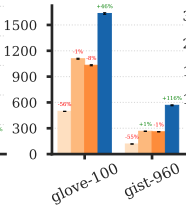
Annoy
