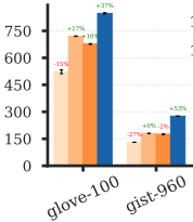
Annoy
