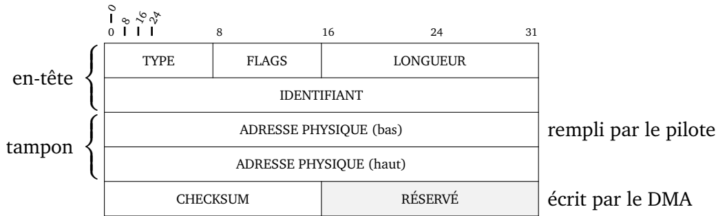
Fig. 2.3: Descripteur d'anneau de réception, avec ses deux groupes de champs.
