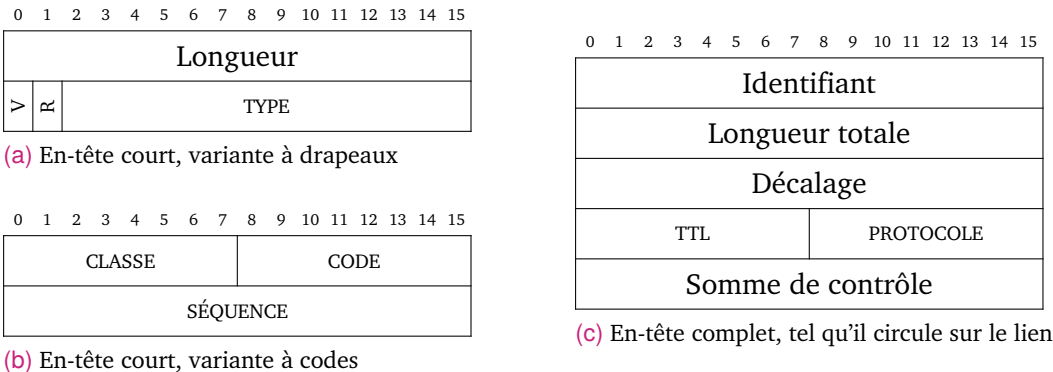
Fig. 2.4: Trois formats d'en-tête, alignés sur la même grille de 16 bits.
