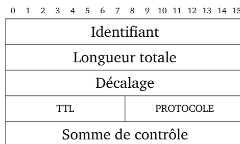
(c) En-tête complet, tel qu'il circule sur le lien
