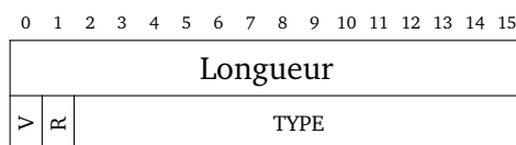
(a) En-tête court, variante à drapeaux
