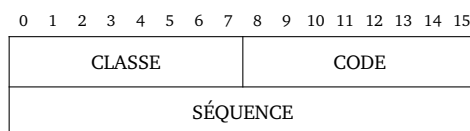
(b) En-tête court, variante à codes
