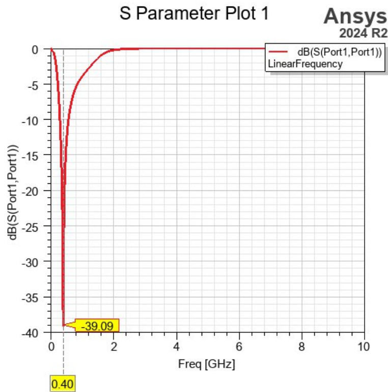
S Parameter Plot 1
