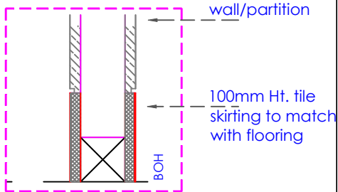
3 SECTION - S3 Scale: 1:4
