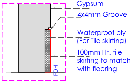
2 SECTION - S2 Scale: 1:4
