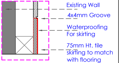
1 SECTION - S1 Scale: 1:4
