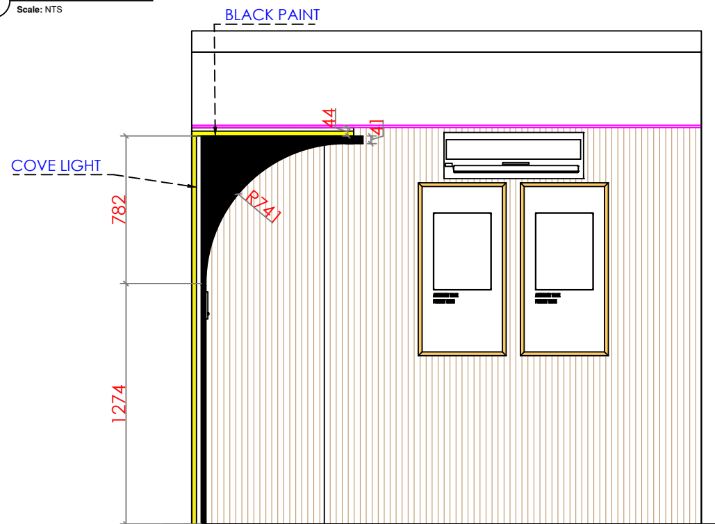
1 ELEVATION E5 Scale: NTS
