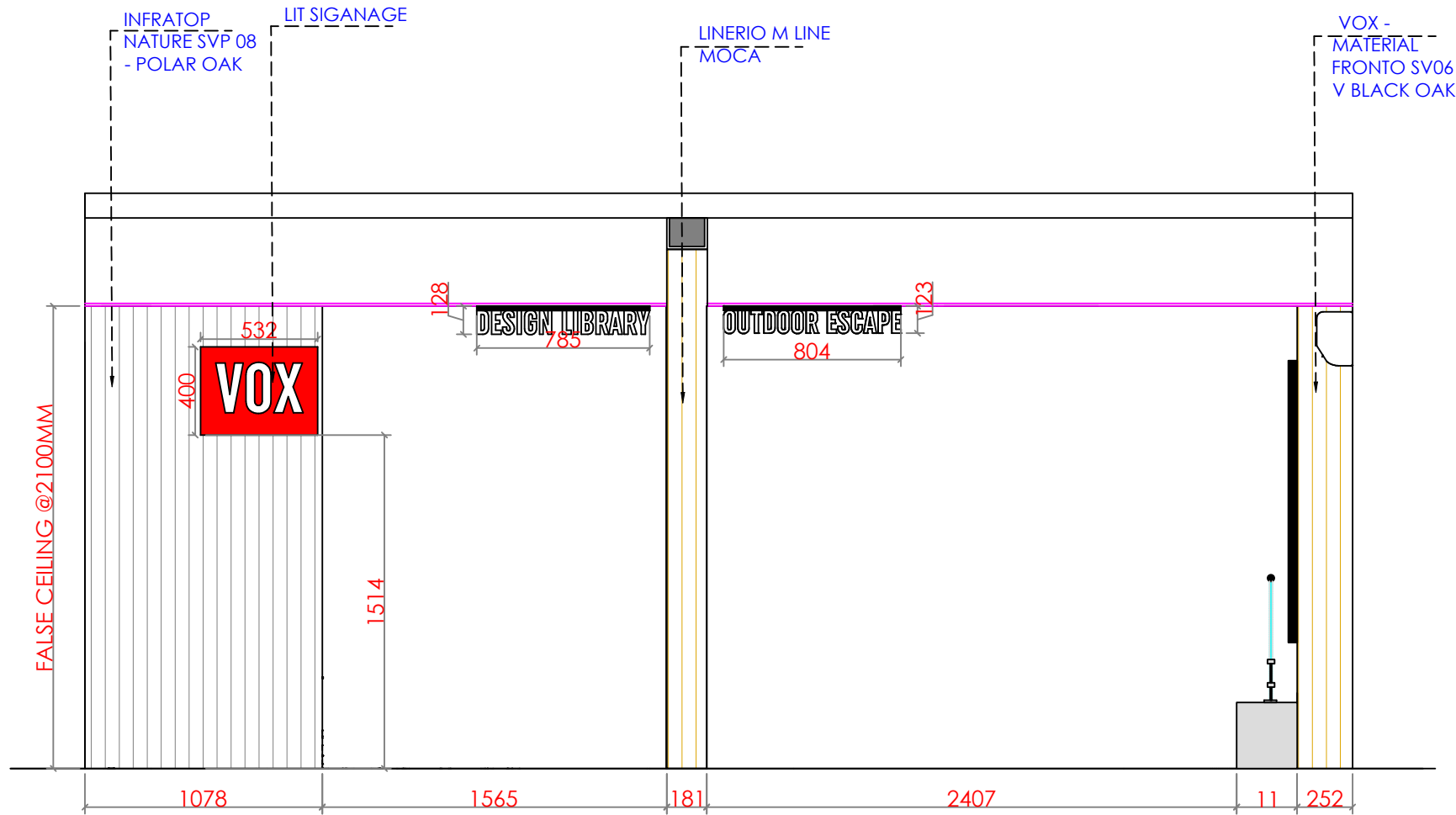
1 ELEVATION E4 Scale: NTS
