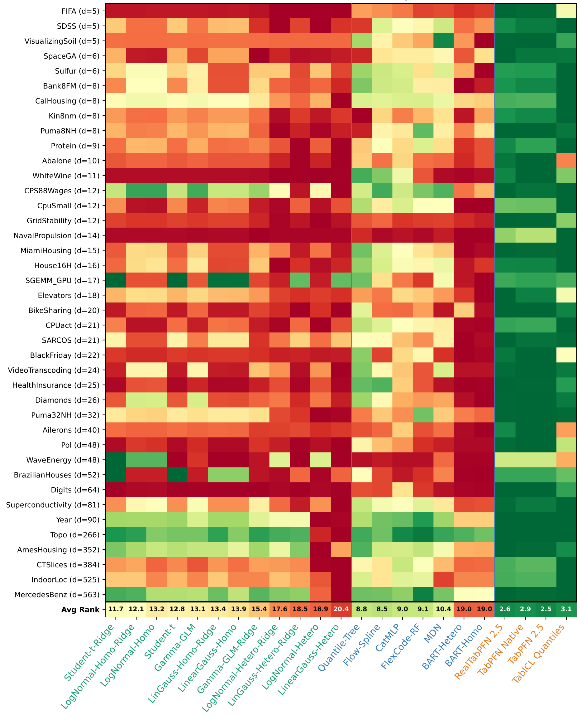
CDE Loss — Raw Values (n=1000, Real)
