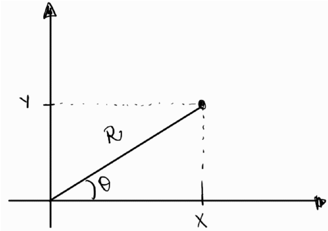
Figure 78.1: Representação em Coordenadas Polares
