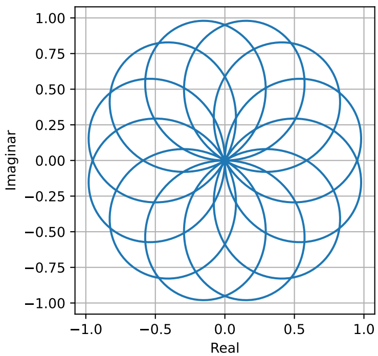
\omega=5
