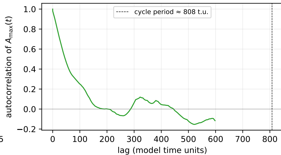
(d) Model A_{\max}(t) autocorrelation (cycle signature)
