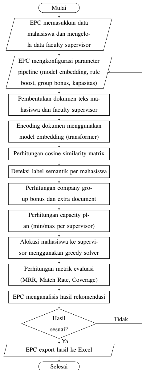
Gambar 3.1. Alur Kerangka Berpikir
