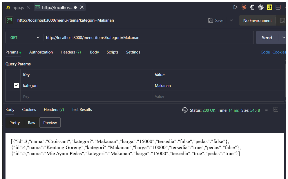
Gambar 4. GET http://localhost:3000/menu-items?kategori=Makanan
