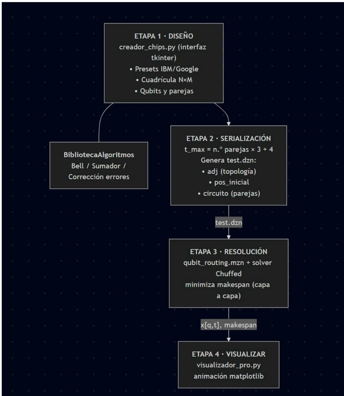
Figura 3.1 — Esquema del sistema: del diseño del chip a la animación del enrutamiento óptimo. El modelo MiniZinc (etapa 3) es el núcleo del trabajo.
