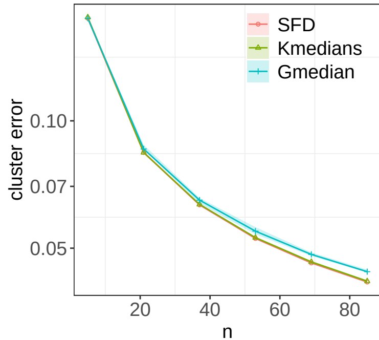
p = 2
