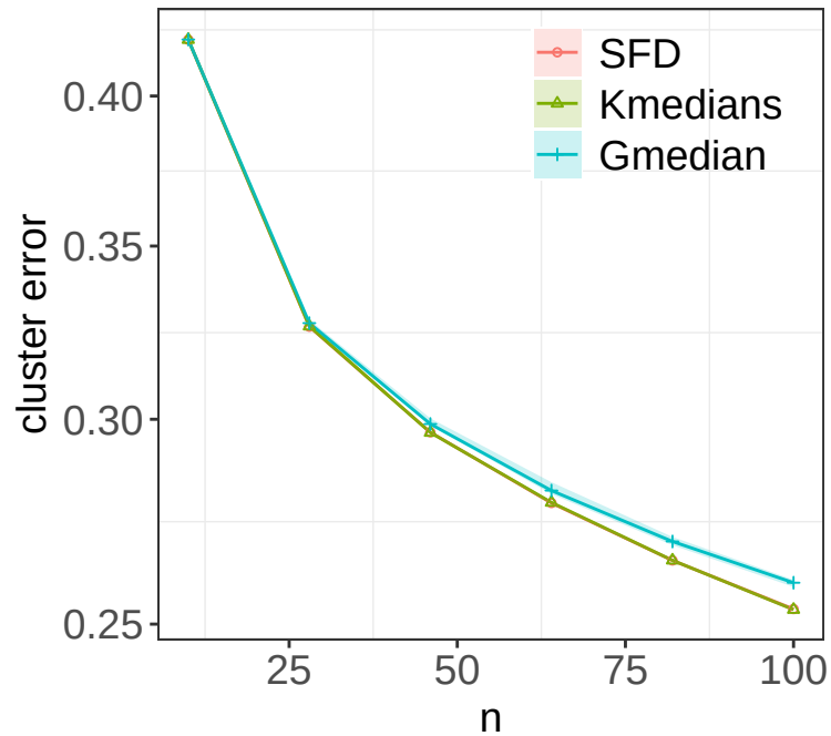
p = 5
