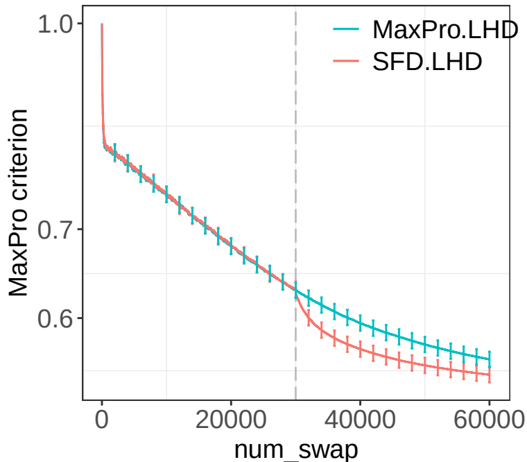
MaxPro Design: p = 10 , n=100
