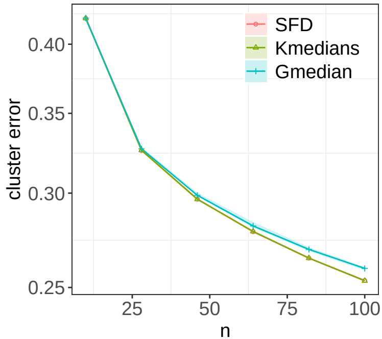
p = 5
