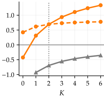
BT MLE estimates
