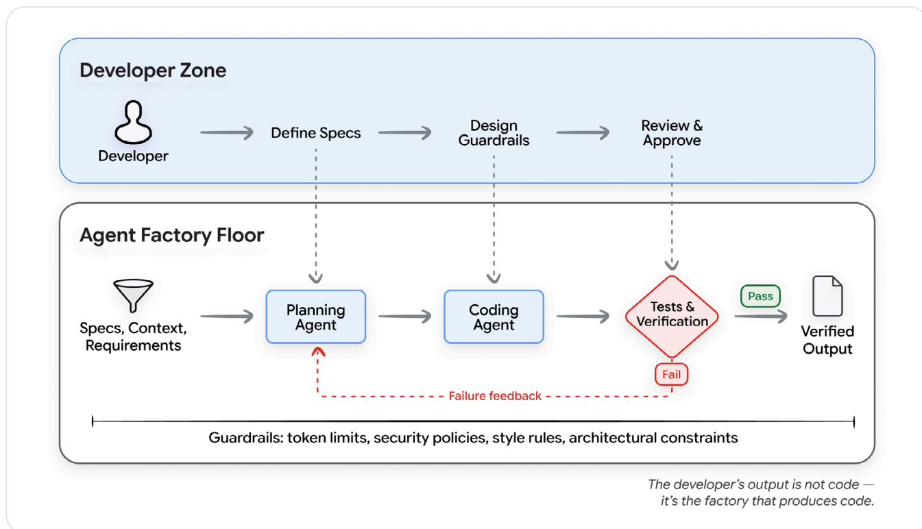
شکل ۶: مدل کارخانه — توسعه‌دهنده سامانه را طراحی می‌کند ← عامل‌ها کد تولید می‌کنند ← تست‌ها خروجی را راستی‌آزمایی می‌کنند.
