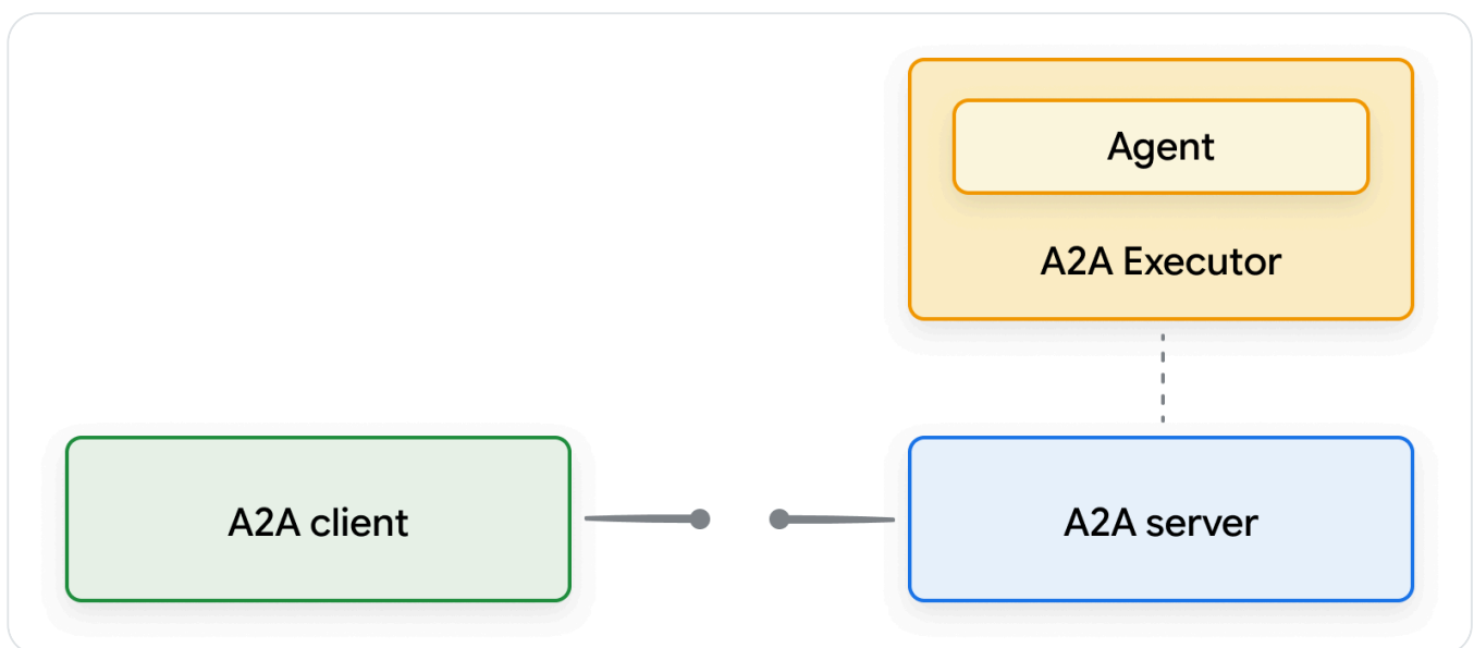
شکل ۵: عرضهٔ سمت‌عرضهٔ یک عامل بومی به‌شکل سرور، و مصرف سمت‌تقاضای آن از راه کلاینت.
