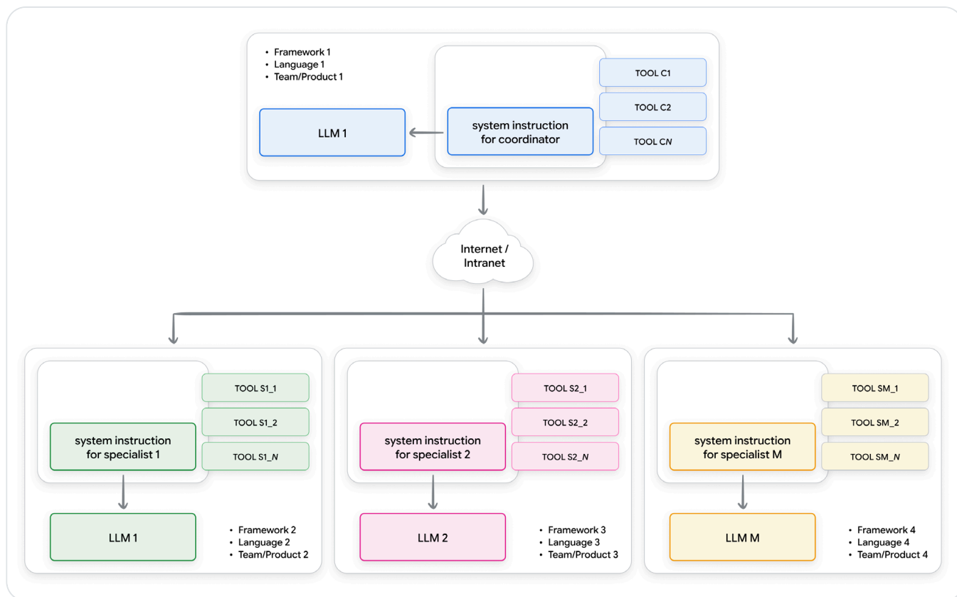
شکل ۴: معماری توزیع‌شده چندعاملی – یک هماهنگ‌کننده کارها را از مرزهای شبکه به عامل‌های راه دور و حوزه‌ویژه واگذار می‌کند.
