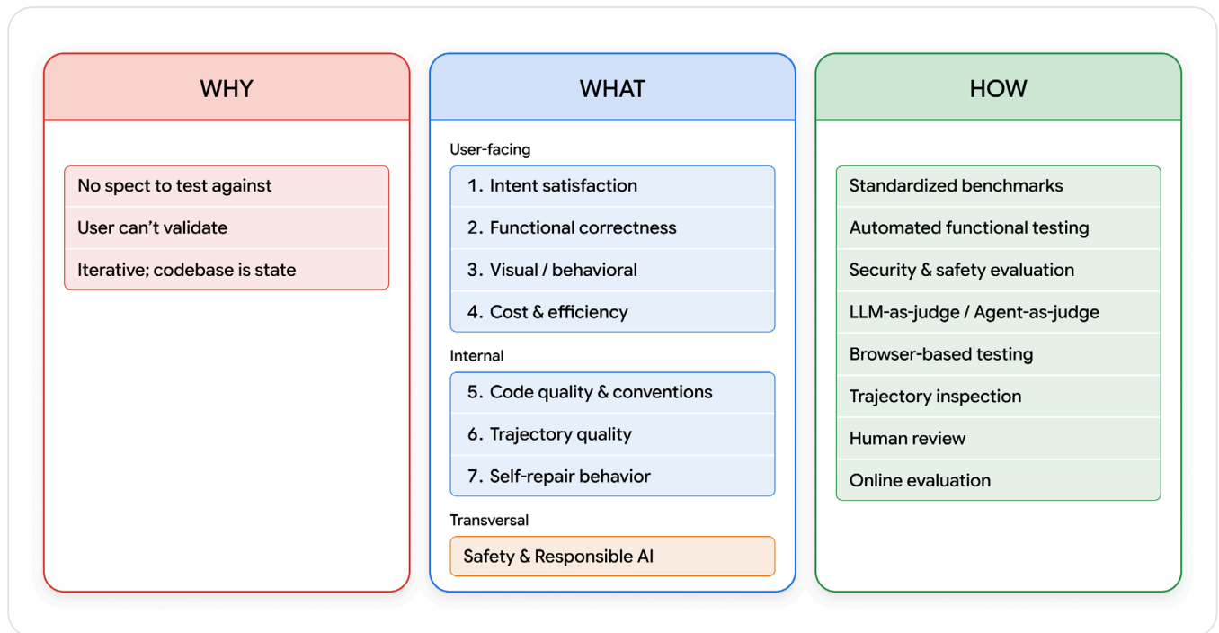
شکل ۲: چراچوب ارزیابی عامل کدنویسی شهودی.
