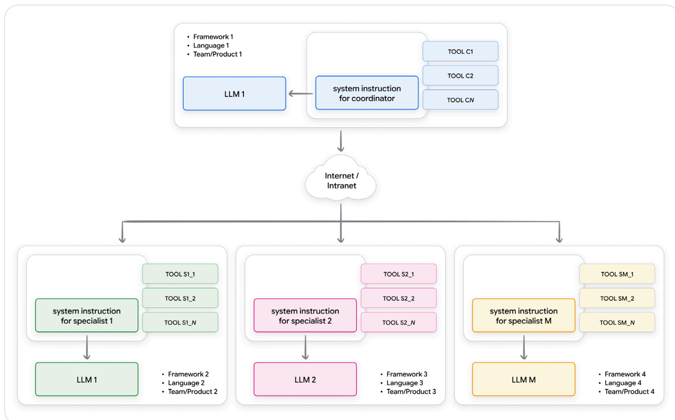
شکل ۴: معماری توزیع‌شده چندعاملی – یک هماهنگ‌کننده کارها را از مرزهای شبکه به عامل‌های راه دور و حوزه‌ویژه واگذار می‌کند.
