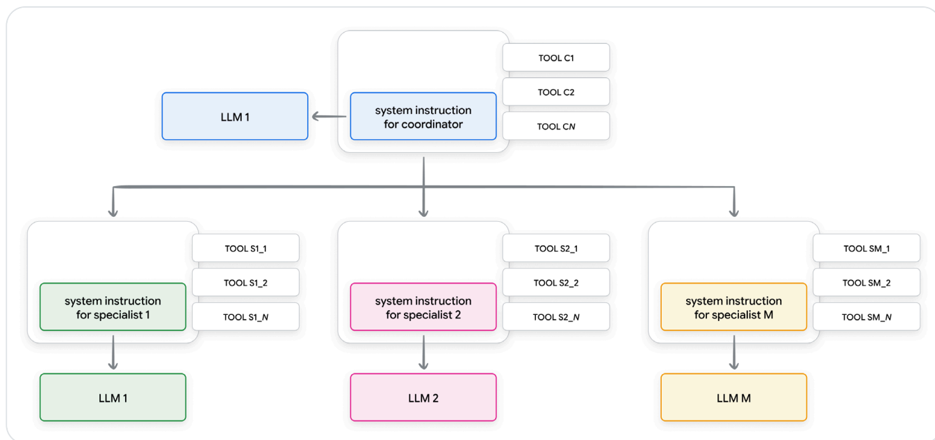
شکل ۳: معماری چندعاملی یکپارچه.
