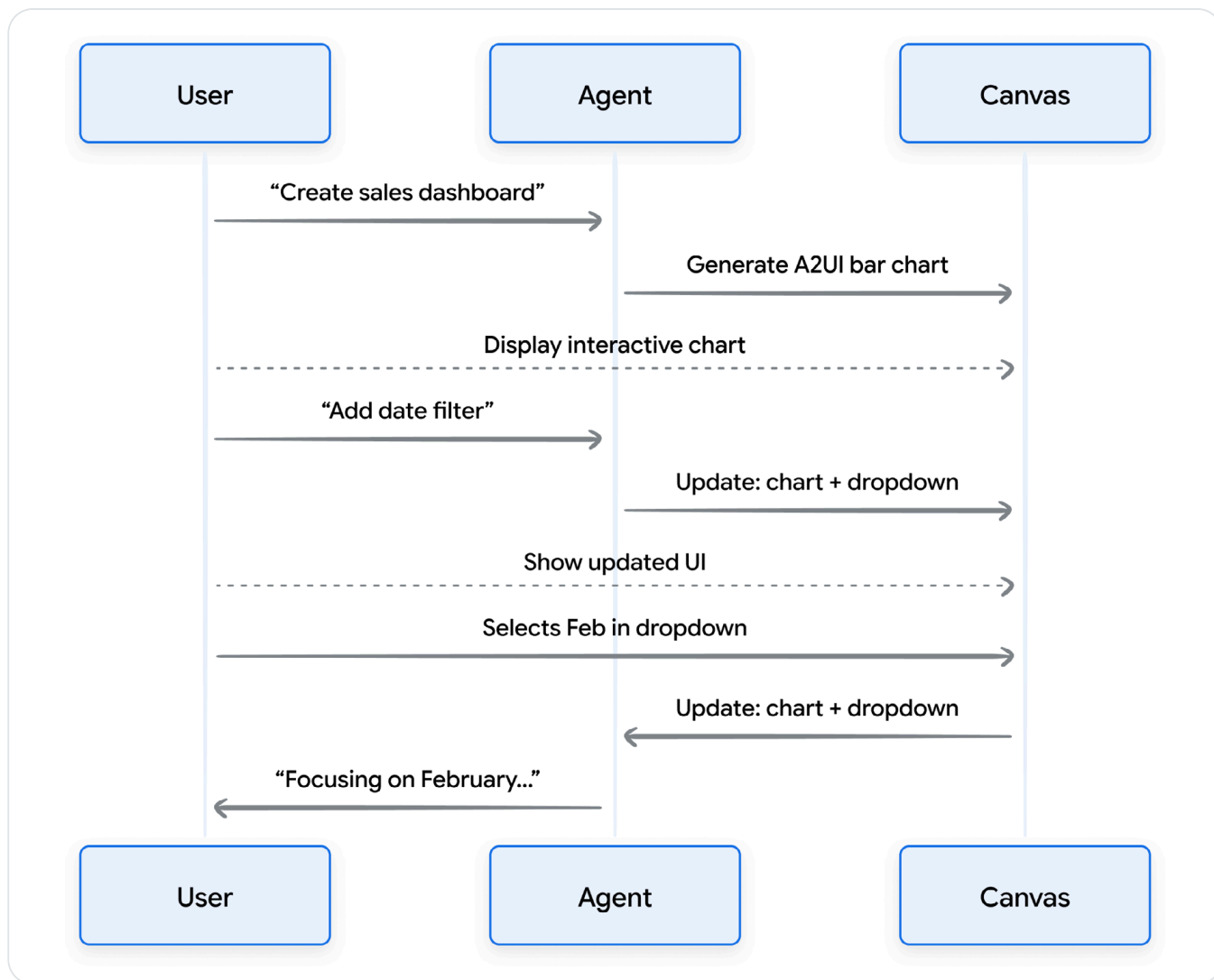
شکل ۷: جریان تعامل کاربر، عامل و بوم. رابط کاربری فقط رندر نمی‌شود؛ رسانه ارتباط است – عامل تعامل‌های شما را مشاهده می‌کند و متناسب پاسخ می‌دهد.
